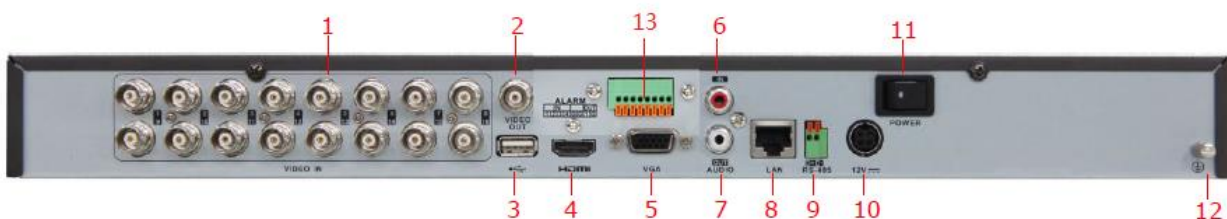
Рис.1.7.3. Задняя панель регистратора LTV-DVR-0861-HV и LTV-DVR-1662-HV
